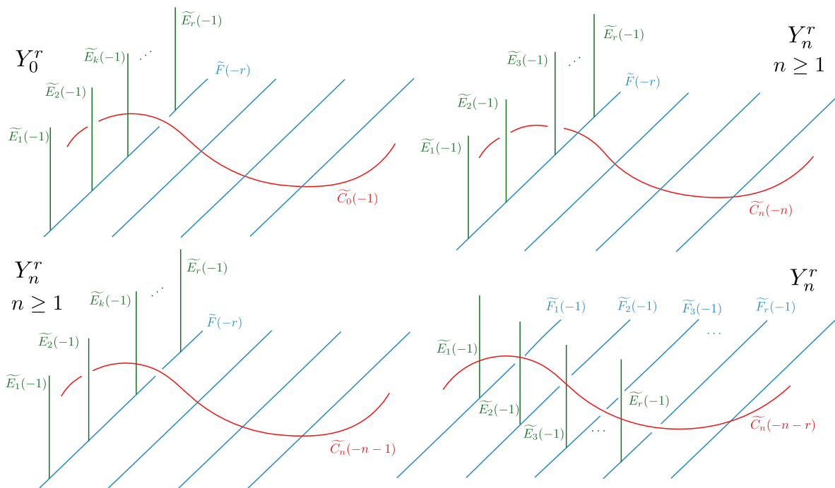
FIGURA 8.2. La superficie Y_n^r .
