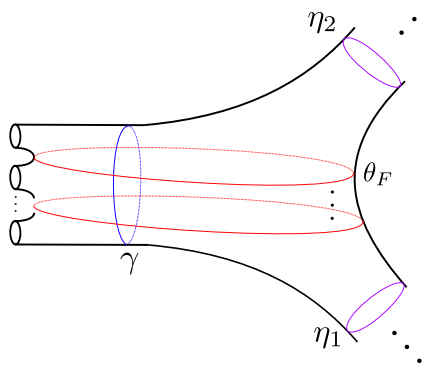
Figura 4.25: Caso b > 1 .
