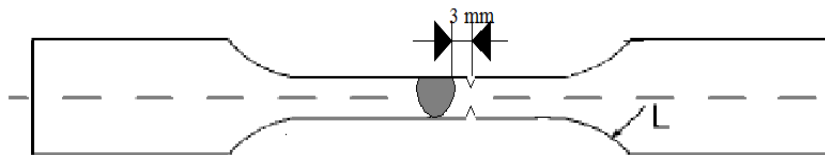
Figura 3. 17 Diseño de la probeta para tensión con muesca de acuerdo a la norma ASTM E338 [40].
