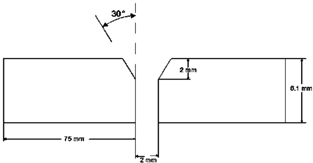
Figura 3. 5 Diseño de la junta en simple “V” en la parte superior.
