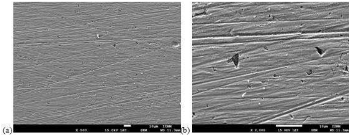
Figura 4. 30 Metal base con tratamiento térmico de envejecimiento en H 2 SO 4 + 0.5M HCl a) 500x y b) 2000x.
