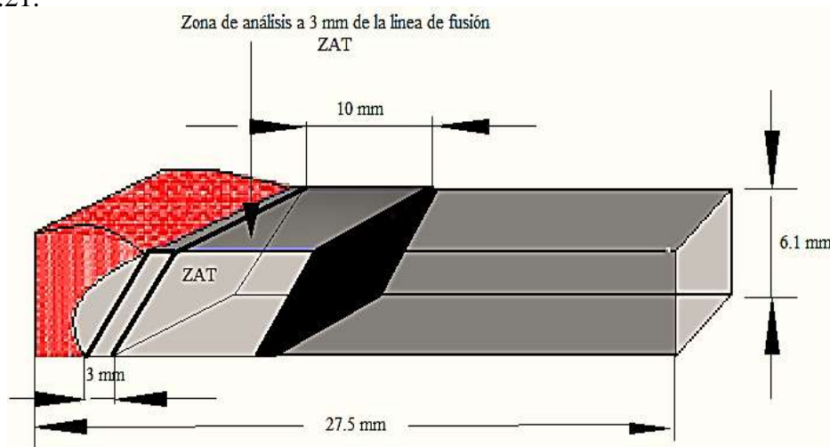
Figura 3. 21 Diseño de la muestra para las pruebas de corrosión.
