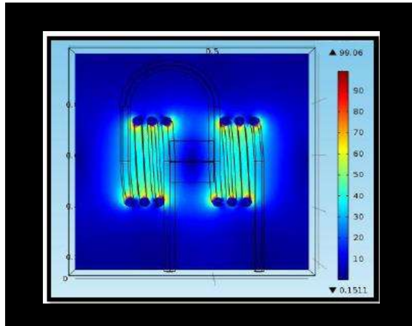
Figura 3. 12 Vista superior de la aplicación de campos magnéticos.
