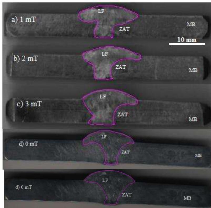
Figura 4. 3 Macrografías de las diferentes condiciones de soldadura.
