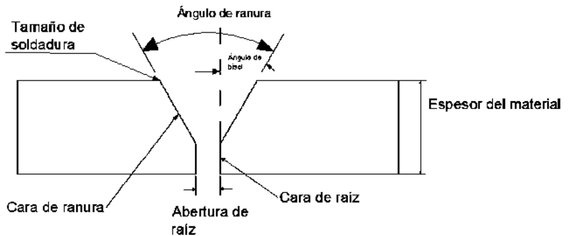
Figura 3. 6 Nomenclatura de una ranura del tipo "V" sencilla.
