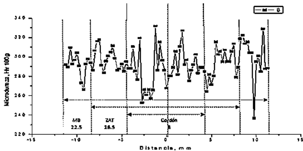
Figura 4. 11 Microdureza del metal base con soldadura convencional.
