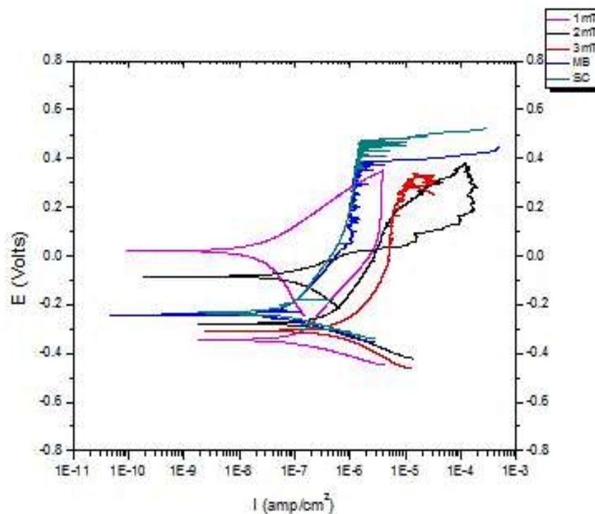
Figura 4. 24 Muestra la tendencia de las curvas de polarización anódica de las condiciones de soldadura.
