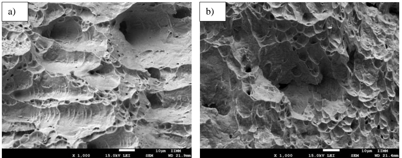
Figura 4. 23 Soldadura con intensidad de campo de 3mT a) 1000x y b) metal base a 1000x.
