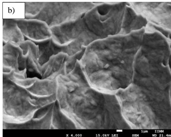
Figura 4. 20 Metal base con muesca a) 1000x y b) a 4000x.
