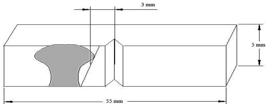
Figura 3. 19 Diseño de la probeta de impacto de acuerdo a la norma E23.
