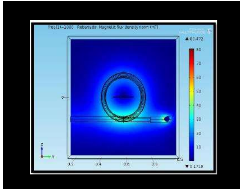
Figura 3.11 Vista lateral de la aplicación de campos magnéticos.
