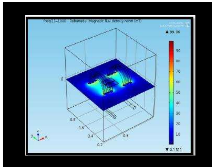
Figura 3. 13 Vista lateral superior de la aplicación de campos magnéticos.
