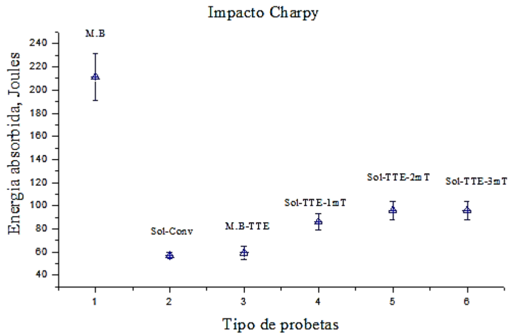
Figura 4. 14 Comportamiento al impacto del acero 316L con las condiciones utilizada en el proyecto.
