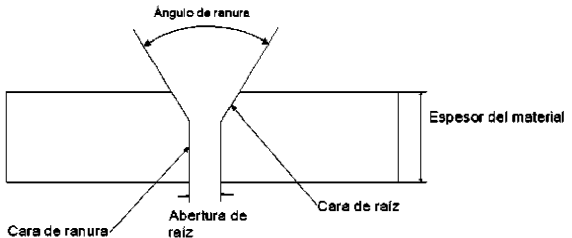
Figura 3. 7 Nomenclatura de una ranura del tipo "V" simple en la parte superior.
