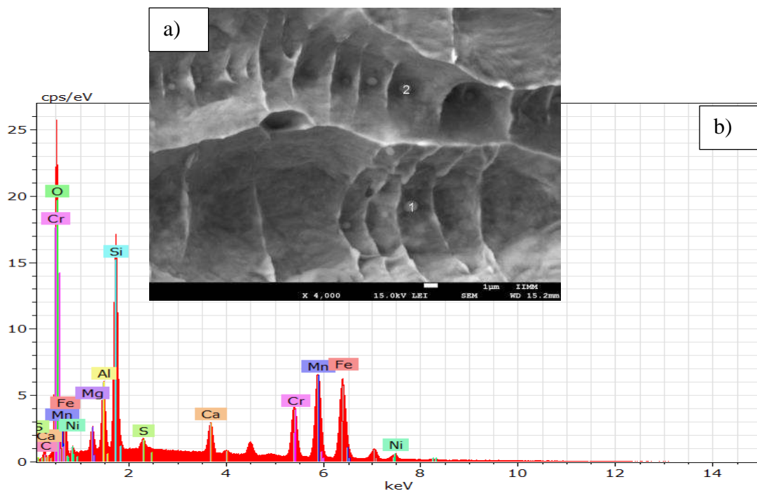
Figura 4. 18 Fractografía de la probeta de 1mT a) 4000x y b) análisis EDS de la figura 4.18 a).
