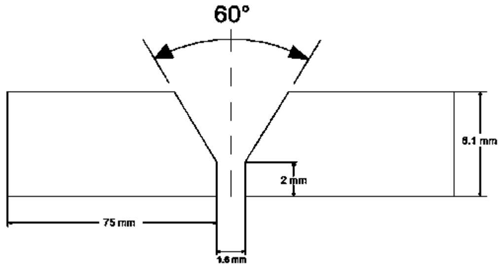
Figura 3. 4 Diseño de la junta en simple “V”.
