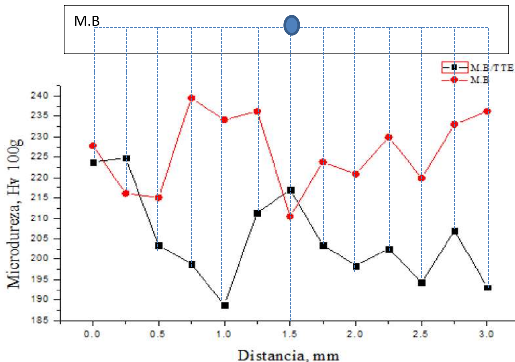
Figura 4. 10 Microdureza del metal base y metal base con TTE sin soldadura ni aplicación de campos magnéticos.
