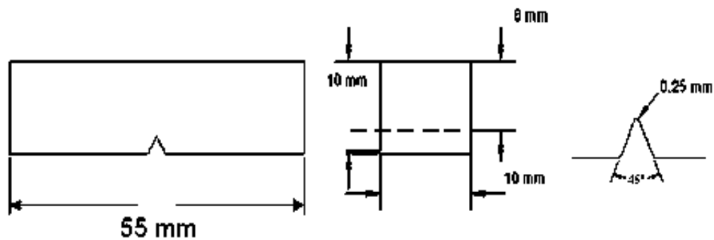
Figura 3. 18 Elaboración de las probetas de impacto tipo muesca, de acuerdo a la norma ASTM E23-56T [41].
