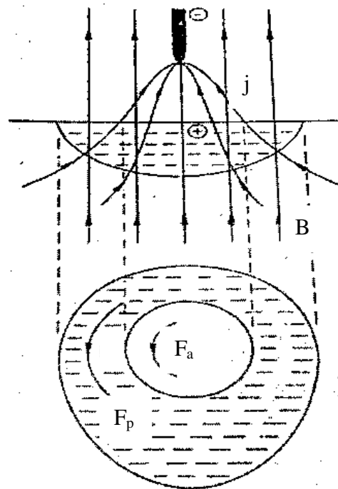
Figura 2. 10 Representación de la influencia de un campo magnético axial en el arco y piletas de soldadura. F_a : fuerza de acción en el arco y F_p : fuerza actuando en la piletas de soldadura [27].
