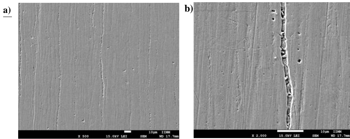
Figura 4. 33 Micrografía de la ZAT de la soldadura con 3 mT (a) 500x y (b) 2000x.
