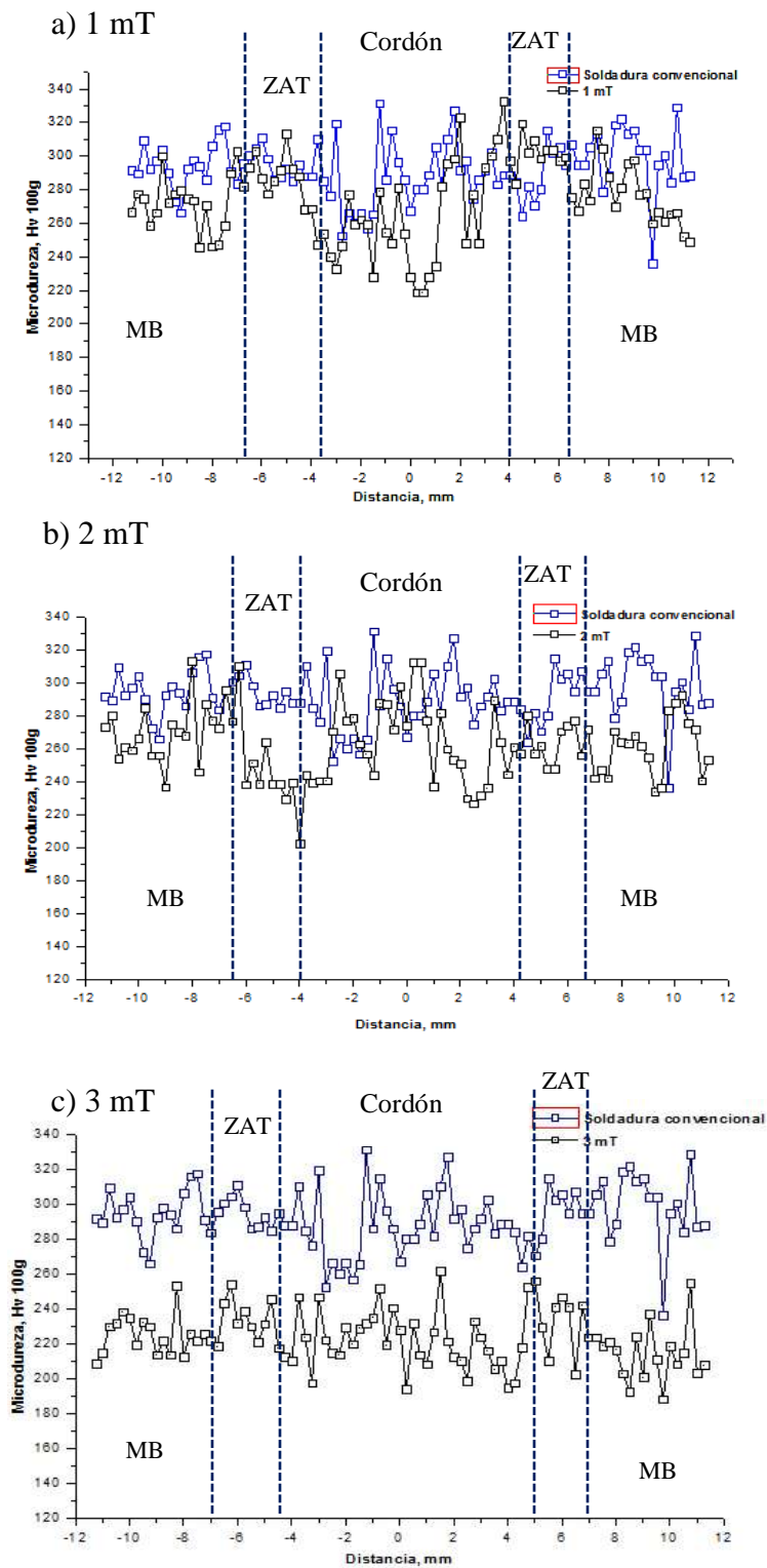
Figura 4. 12 Perfiles de microdureza en las distintas condiciones de soldadura; a) 1 mT, b) 2 mT y c) 3 mT.
