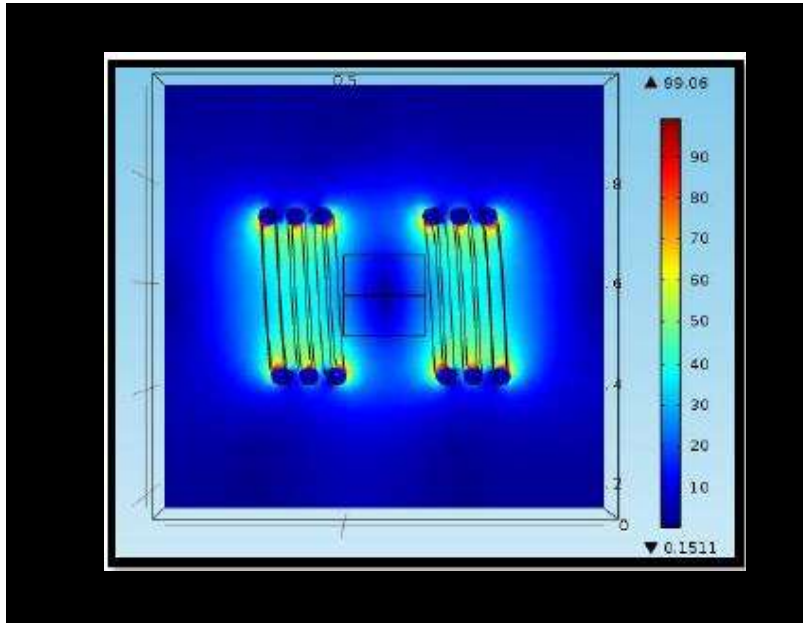
Figura 3.10 Vista superior de la forma de la interacción electromagnética durante el proceso de soldadura. Simulación utilizando software COMSOL Multiphysics®.
