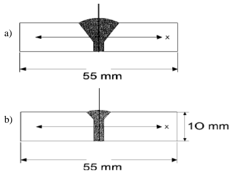
Figura 3. 20 Representación esquemática de la forma en que se realizó el barrido para la obtención de la microdureza: a) soldadura convencional y b) soldadura con TTE e interacción electromagnética.
