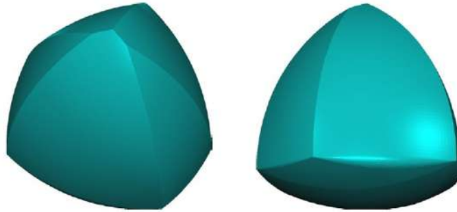
Figura 3.4: Un cuerpo de ancho constante obtenido de un pentágono de Reuleaux.
