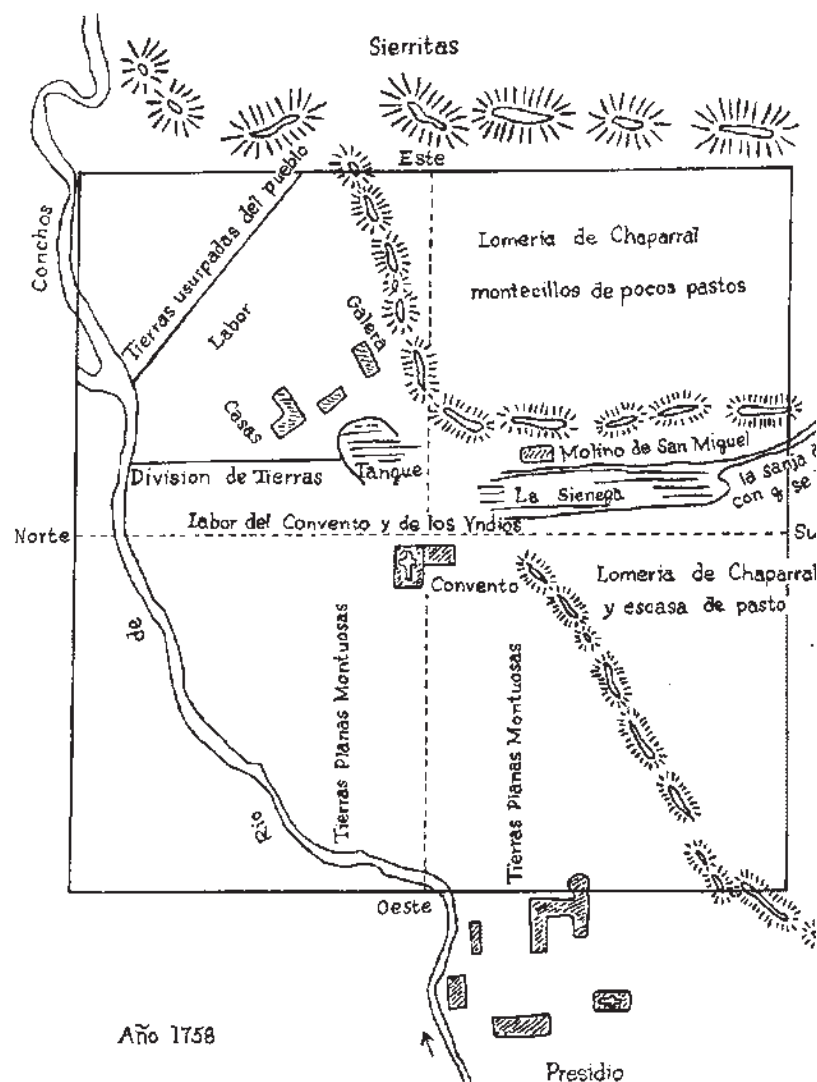
Fig. 3.16.-Plano en el que aparece el presidio de San Francisco de Conchos, que fue localizado en la presidencia municipal del pueblo. 149 Se muestra un conjunto de cinco edificios dibujados por abajo de la línea que dice Oeste. Nótese que la línea horizontal de abajo, pasa por encima de un edificio con un extremo redondeado que es la representación de una torre que resguarda el conjunto; nos permitimos suponer que los rectángulos más alejados que están junto al río deben ser depósitos de material peligroso, quizás polvorines. Por su tamaño, creemos que el rectángulo más grande, que está abajo del edificio principal debe ser la caballeriza y el establo que requerían mucho espacio, mientras que el rectángulo que muestra una cruz representa la capilla.
