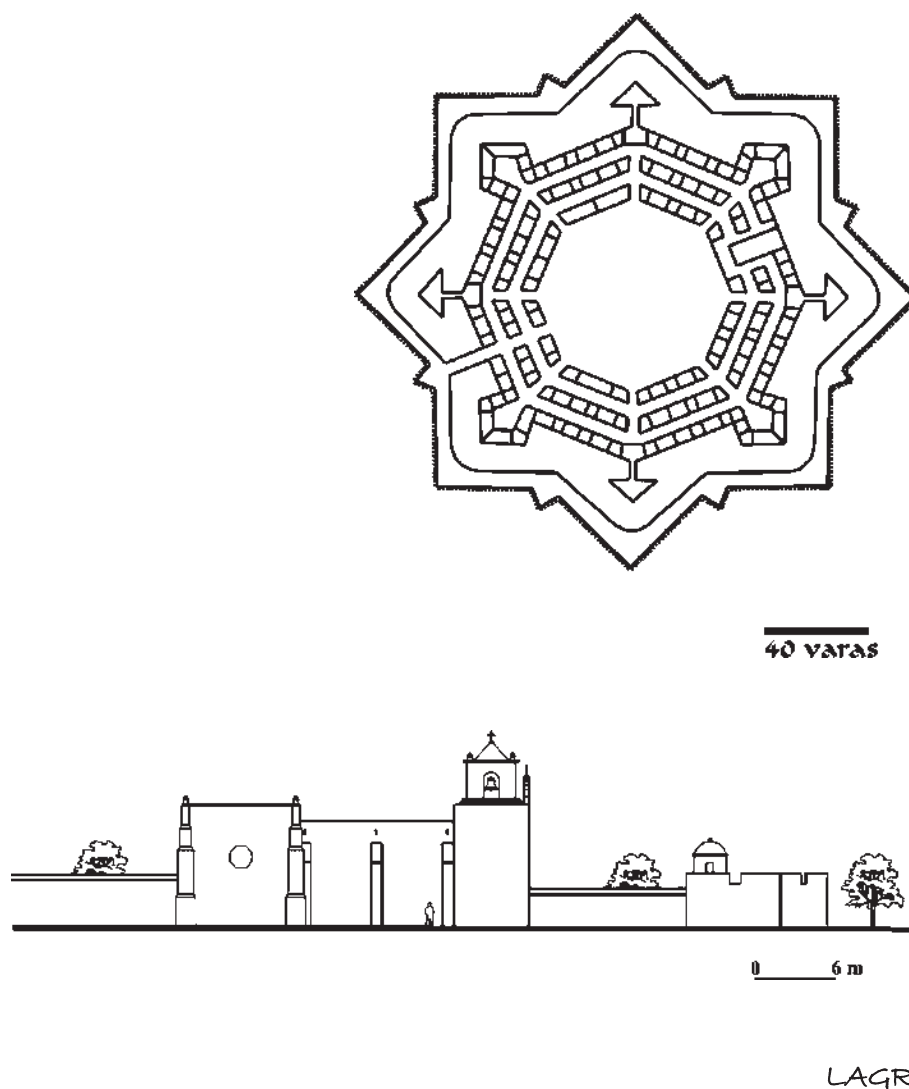
Fig. 4.13.-Arriba: Plano del presidio de Nuestra Señora de Loreto de la Bahía del Espíritu Santo, de 1722, 141 es un conjunto de planta poligonal que no fue terminado. Abajo: Apunte de una sección de la muralla y del testero del templo, que fueron hechos con mampostería. Este presidio ha sido cuidadosamente restaurado y se conserva en Goliad, Texas. A la derecha puede verse un garitón que sobresale por arriba de la barda, junto a un bastión que protege desde la esquina. 142
