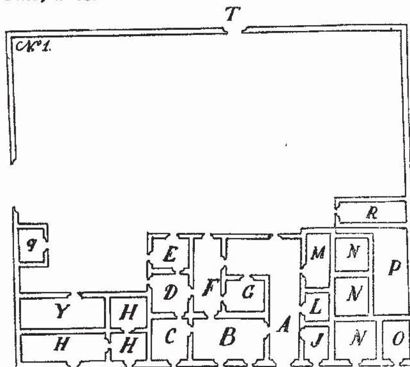
Fig. 4.7.-Plano de la Casafuerte que albergó al presidio de Santa Rosa María del Sacramento. A.-Zaguán, B.-Sala, C.-Recámara, 1a, 2.-Recámara, 2a, E.-Cuarto de criados, F.-Secretaría, G.-Despacho, H.-Cuartel viejo de la Compañía de la Babia, I (Bodega en que está encerrada la madera, J.-Cuarto de la guardia, K.-Despensa, M.-Cocina, N.-Tres cuartos sin techo, O.-Cuarto destinado para la Artillería, P.-Un cuarto sin correspondencia a la sala, R.-Jacal, S.-Patio, T.-Huerta recientemente cercada de adobe. 88
