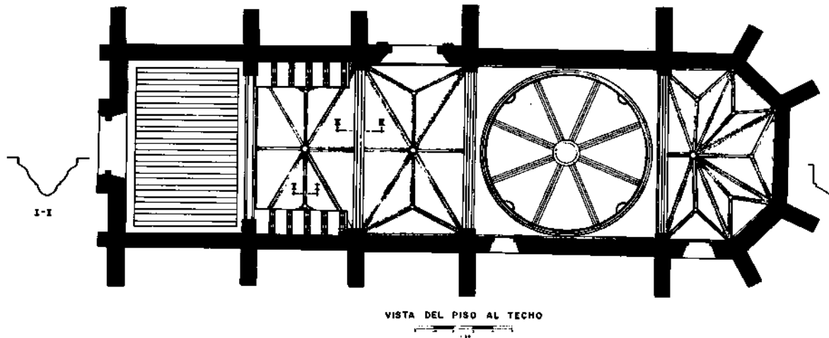
Figura 4.56. Planta de la Iglesia de Regina Angelorum.
