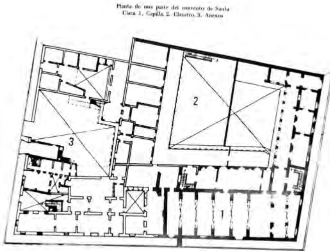
Figura 4.60. Planta Convento e Iglesia de Santa Clara.
