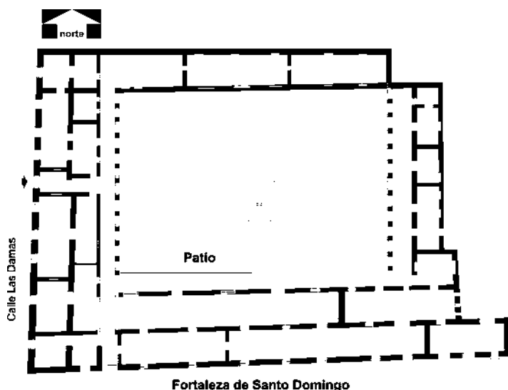
Figura 4.97. Plano Casa de Bastidas.
