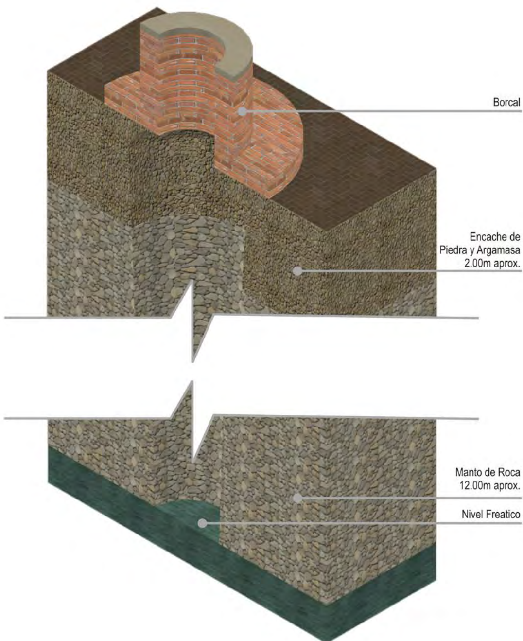
Figura 4.129. Esquema Tipológico de Pozos Excavados. Aportación de la autora basada en entrevista con el Lic. Fransisco Coste , Encargado del Departamento de Arqurología. Dirección Nacional de Patrimonio Monu- mental. Santo Domingo, Noviembre, 2006. Modelo Digital e Infografía: Jorge Marte.
