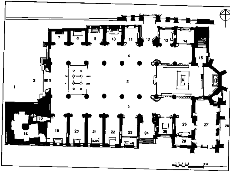
Figura 4.52. Planta Catedral Santa María de la Encarnación. Plano: Dirección Nacional de Patrimonio Monumental.
