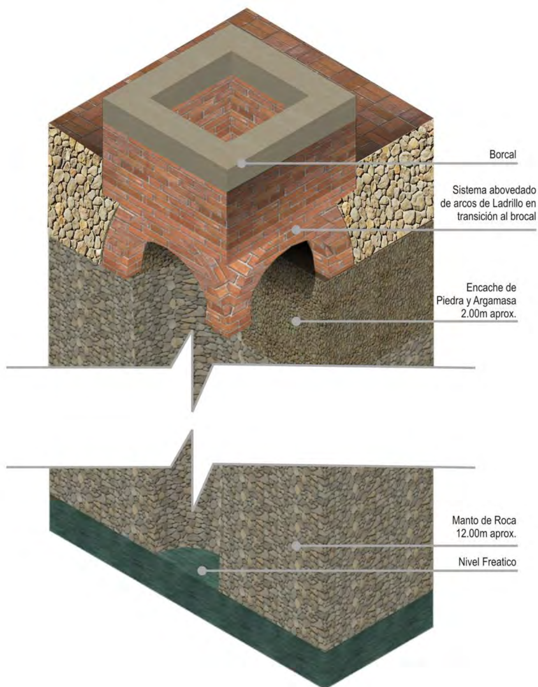
Figura 4.130. Esquema Tipológico de Pozos Excavados con Bóvedas de Transición al Brocal. Aportación de la autora basada en entrevista con el Lic. Francisco Coste , Encargado del Departamento de Arqueología. Dirección Nacional de Patrimonio Monumental. Santo Domingo, Noviembre, 2006. Modelo Digital e Infografía: Jorge Marte.
